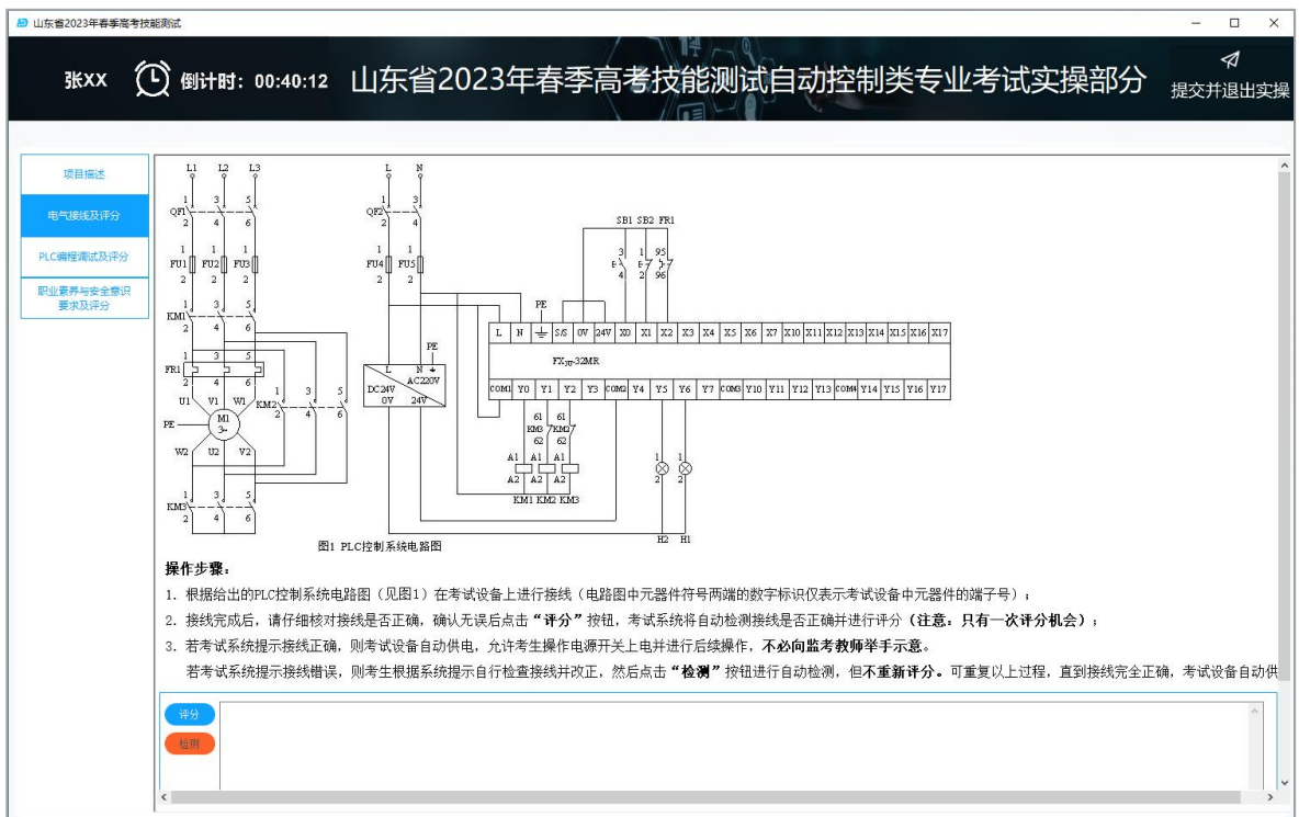
图7 实操部分-电气接线及评分界面
